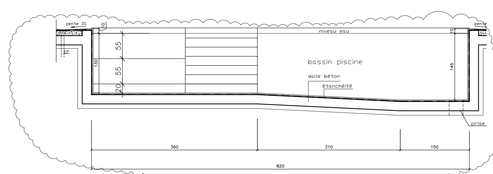
COUPE LONGITUDINALE SUR PISCINE ECH. 1/50
